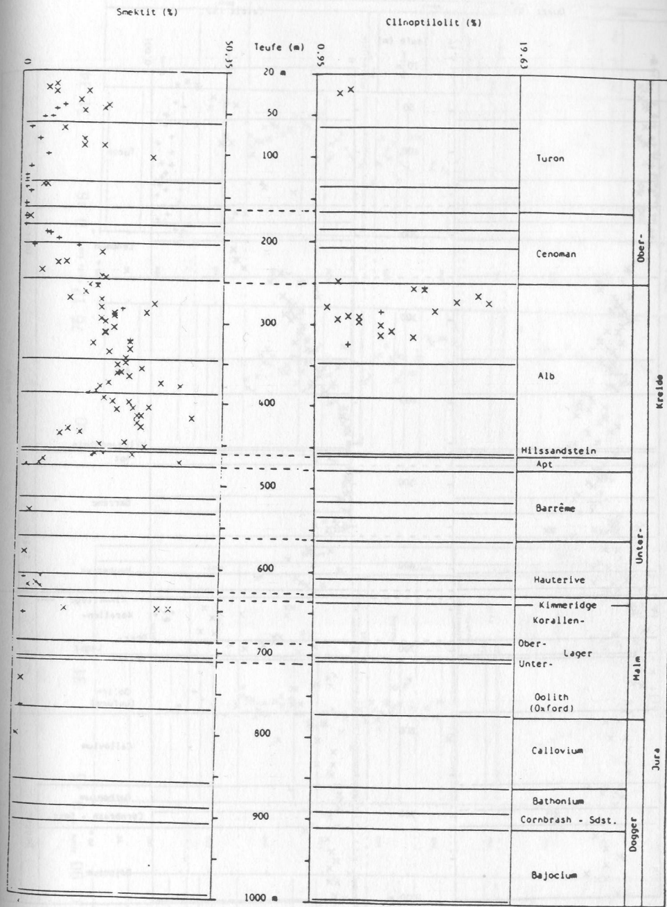
Abb. 11: Verteilung von Smektit und Klinoptilolith im Profil der Bohrung Konrad 101 (BGR, 1989)
