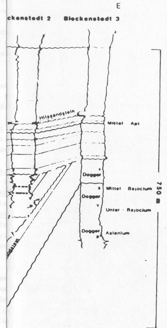
Abb. 9: Profil der Bohrung Konrad 101 im Vergleich zu benachbarten Bohrprofilen (BGR, 1990)
