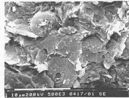
b) Mittelbarrême; parallel zur Schichtung; Coccolithen-Lage in toniger Matrix
