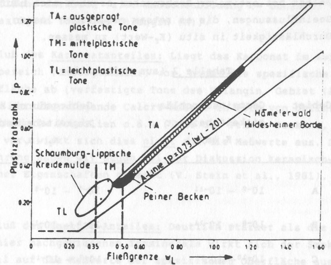
Abb. 8: Plastizitätsbereich der untersuchten Tongesteine (nach DIN 18196). (Aus: NLFb, 1986)
