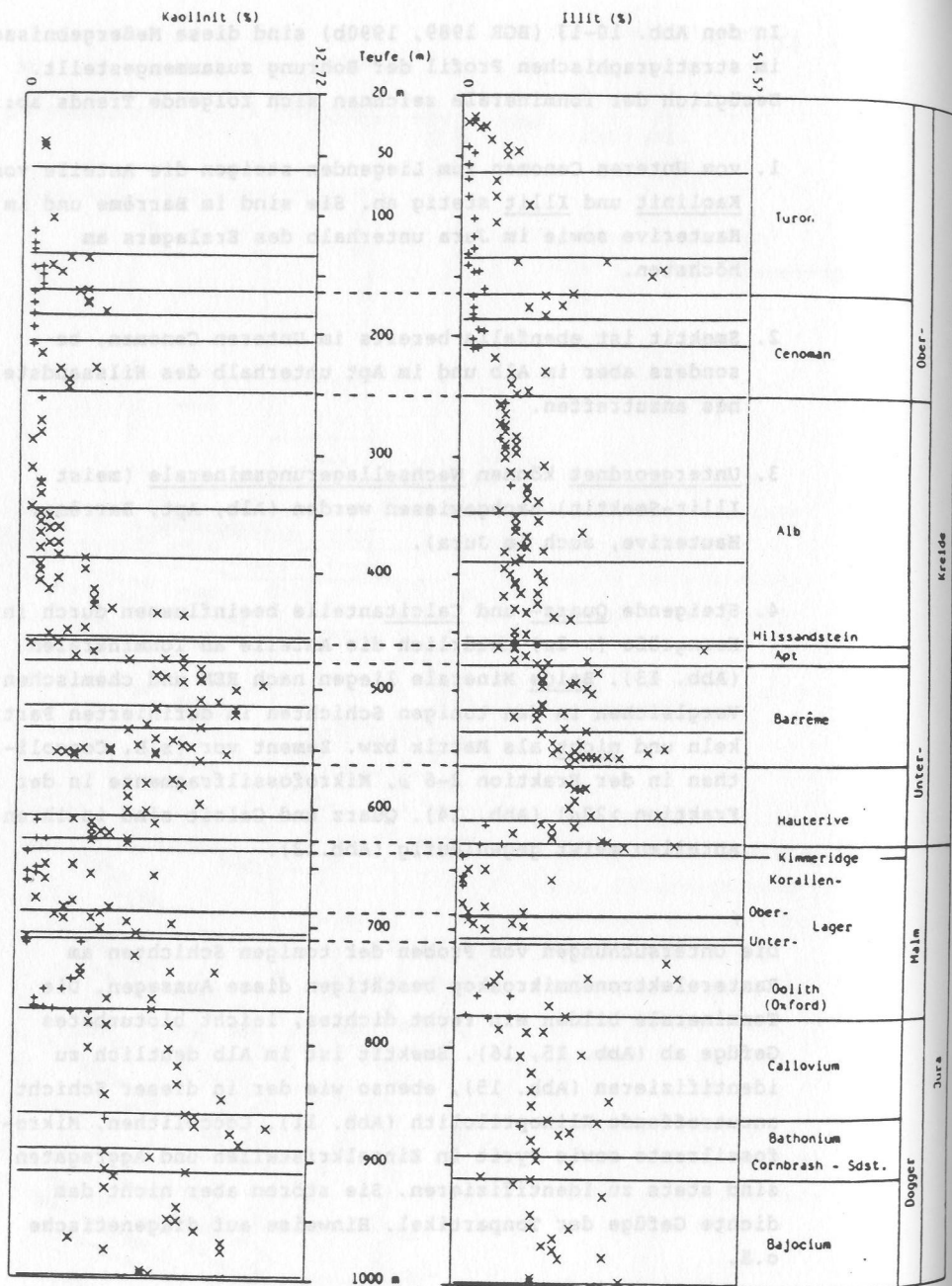
Abb. 10: Verteilung von Kaolinit und Illit im Profil der Bohrung Konrad 101 (BGR, 1989)
