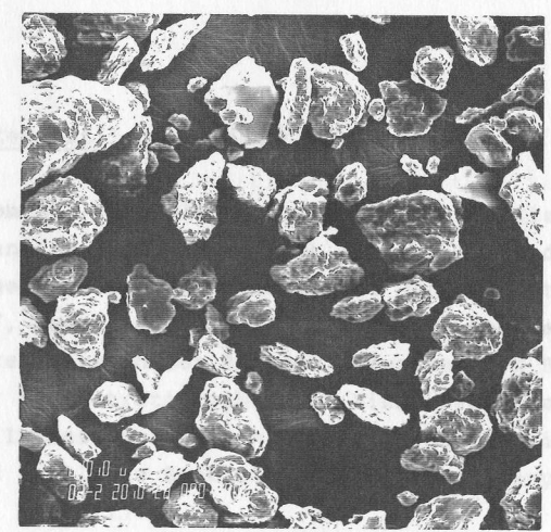
b) ausgelesene calcitverkrustete Tonaggregate ("Knötchen")
