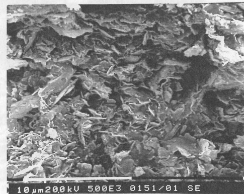
a) Oberalb: feinkörniger Smektit neben Tonpartikeln
