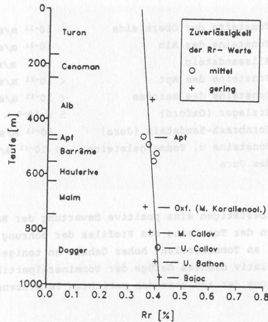
Abb. 17: Inkohlung Bohrung Konrad 101
