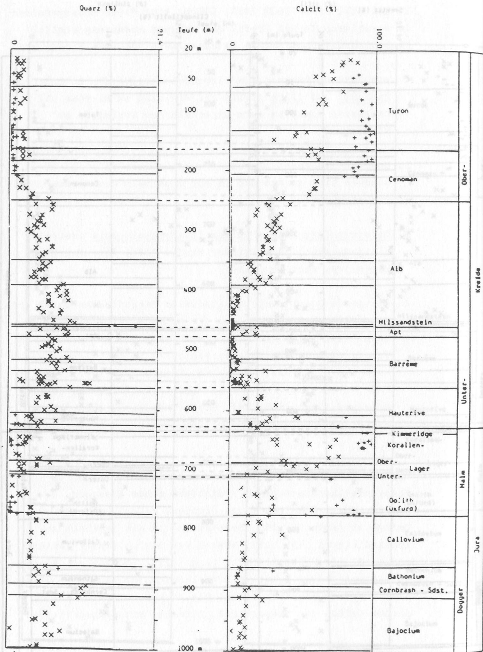
Abb. 12: Verteilung von Quarz und Calcit im Profil der Bohrung Konrad 101 (BGR, 1989)
