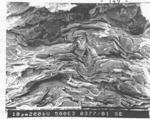
a) Oberbarrême; senkrecht zur Schichtung; im Zentrum ein Pyrit-Kristall
