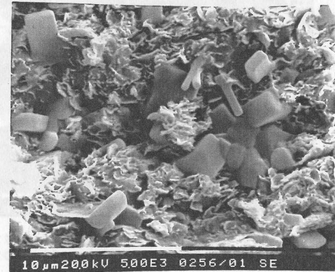
b) Unteralb: wie Abb. 14a, NaCl-Kristalle aus Porenwasser
